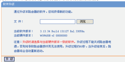
图2-81 软件升级
